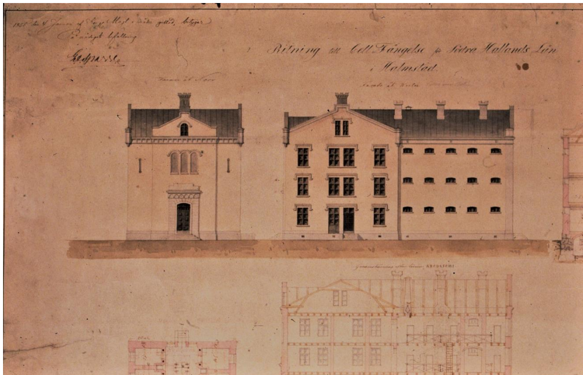
Denna och föregående sida: Utsnitt av nybyggnadsritning ritad av T.h. Ankarsvård undertecknad av C F Hjelm, Stockholm den 29 september 1854 och gillad av Kongl Majt den 4 januari 1855. Notera att den västra fasaden har bytt plats med den östra på den färdigställda byggnaden.
