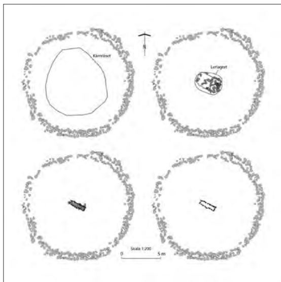
4. Planerna visar de olika konstruktionselementen i gravhögen.
