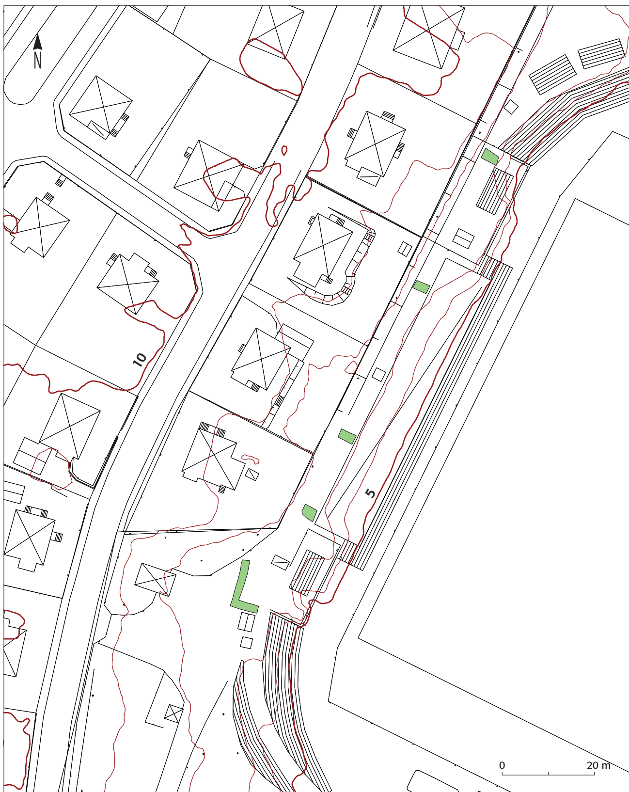
Fig 2. Grävningstorna fanns inom ett område där markytan låg på mellan 7 och 8 meter över havet. Skala 1:800.
