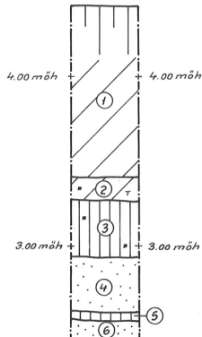
SEKTION 15, SSV
