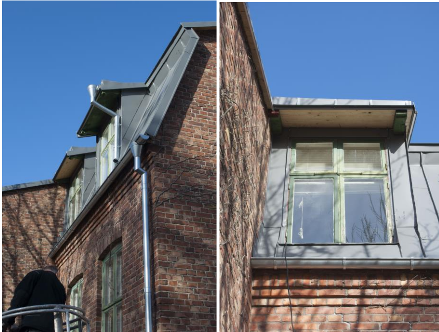
En stor del av råsponten fick bytas på gårdshuset, vilket syns på undertaket på ena takkupan.
