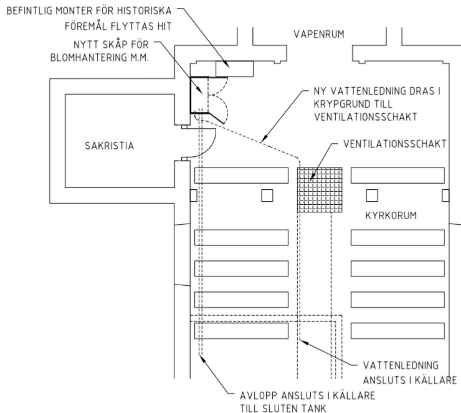
Figur 2. Del av plan för Dagsås kyrka.
