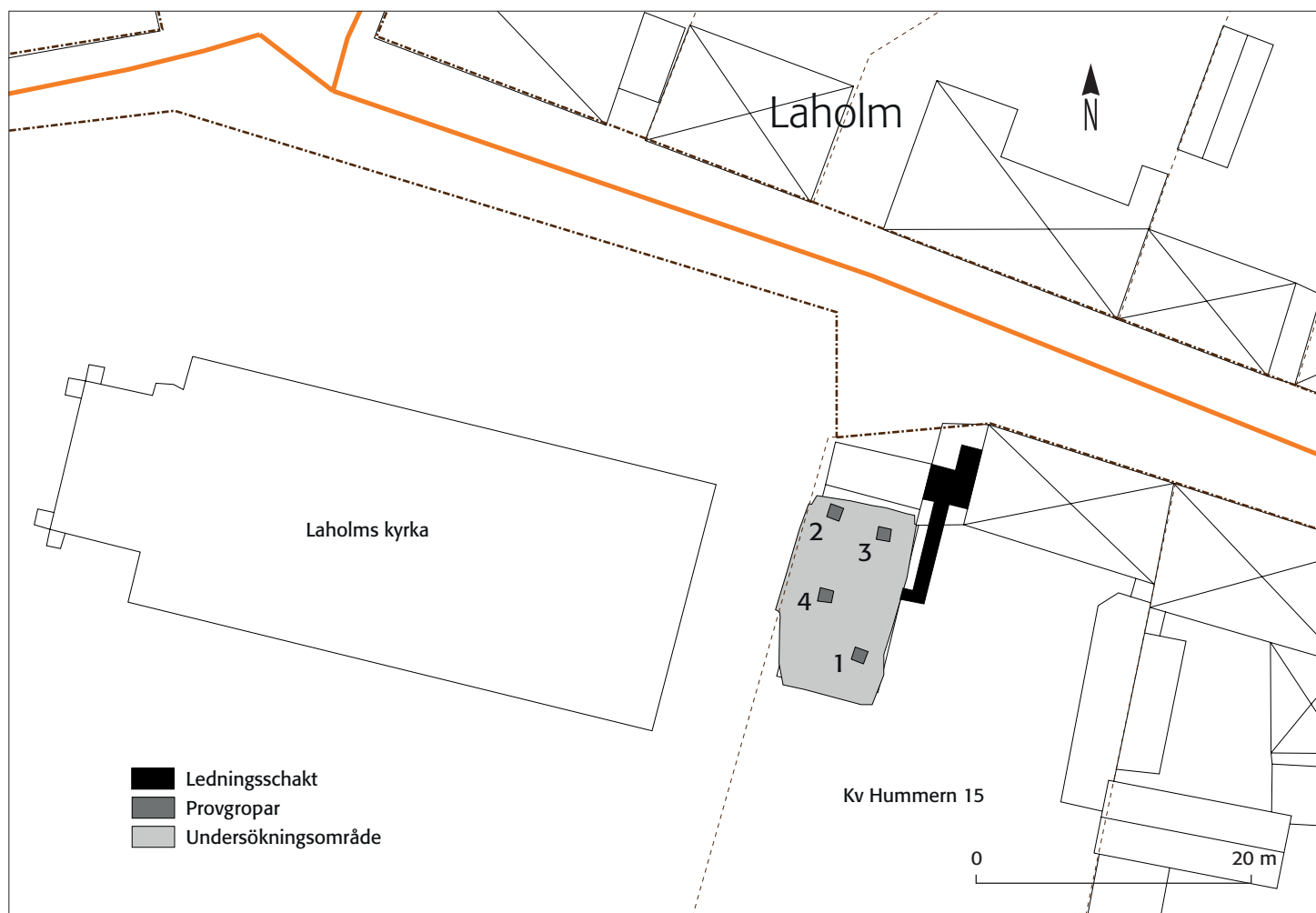
Figur 3. Karta över undersökningsområdet med ledningsschakt och provgropar markerade. Skala 1:500.
